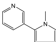
Nicotine
