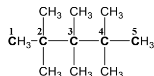
2,2,3,3,4,4-Hexa methyl pentane
