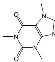
Caffeine
