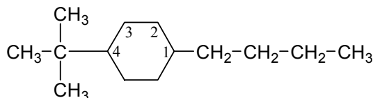
1-n-Butyl-4-tert-butyl cyclohexane
