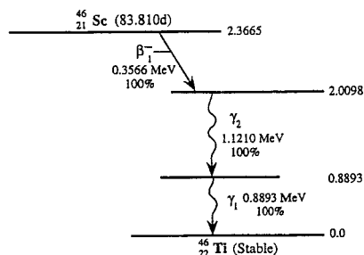
45 Sc(n, γ) (Apr. 28, 1993)
